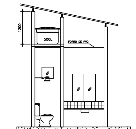
CORTE "C-C"
