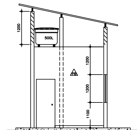
CORTE "B-B"
