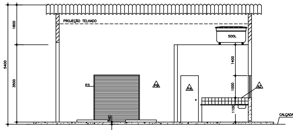
CORTE "A-A"
